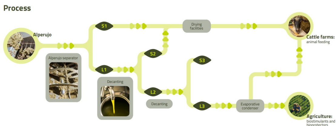
Figura 1 Proceso definitivo de separación de alperujo
